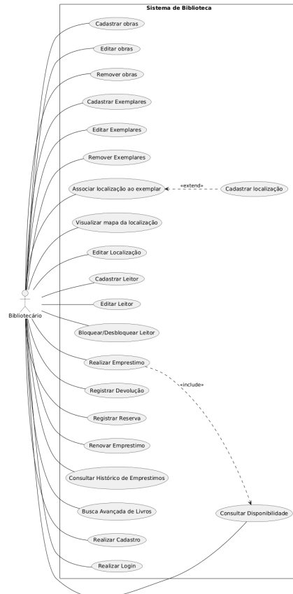
Figura 1 – Diagrama de Casos de Uso: Módulo Bibliotecário
