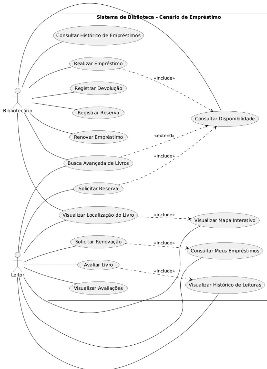
Figura 3 – Diagrama de Casos de Uso: Cenário de Empréstimo
