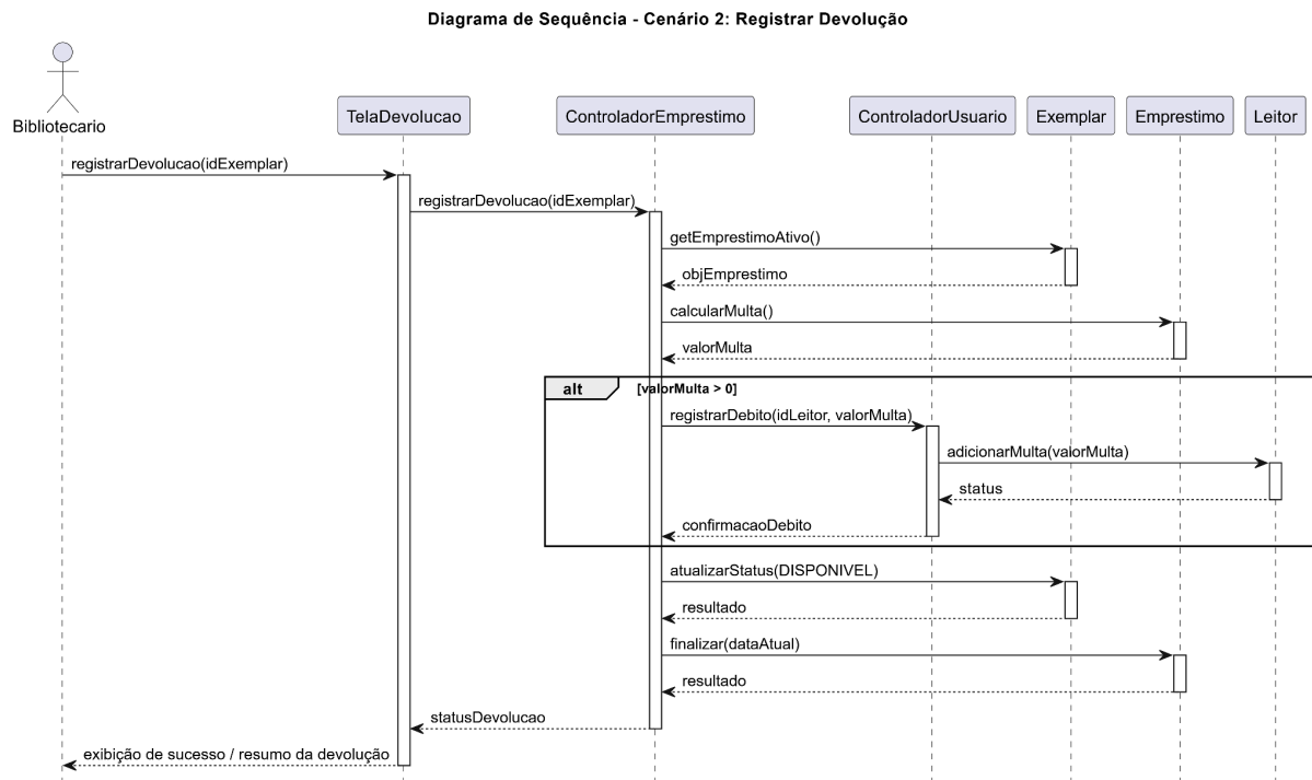
Figura 6 – Diagrama de Sequência: Cenário de Realizar Devolução
