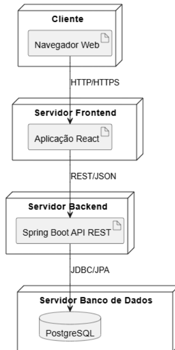
Figura 7 – Diagrama de Implantação
