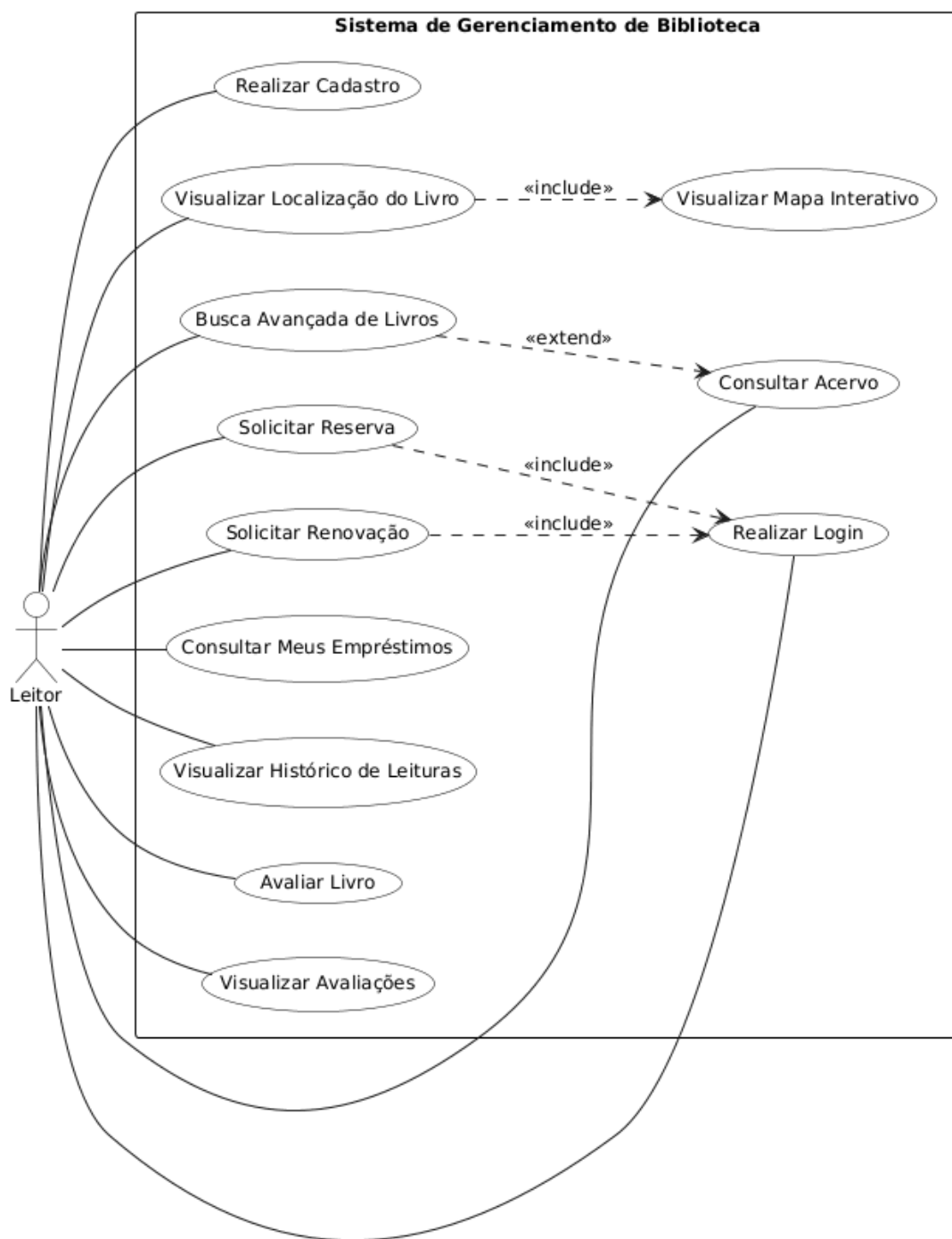
Figura 2 – Diagrama de Casos de Uso: Módulo Leitor
